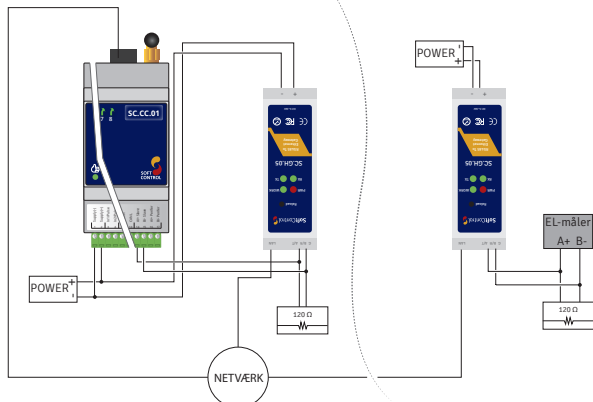
Ill. 2 - Illustration af diagram ift. montering af Modbus el-måler.
