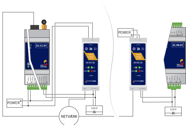
Ill. 4 - Illustration af diagram ift. montering af varmestyring vha. SC.IM.01.
